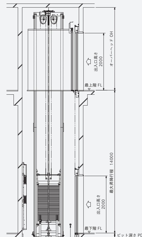
昇降路断面図
