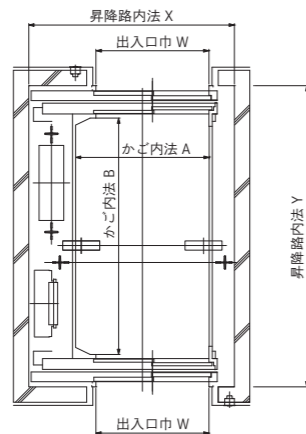
昇降路平面図
