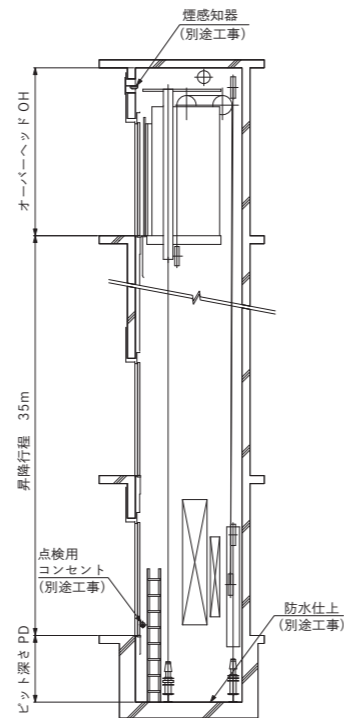
昇降路断面図
