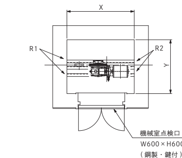
機械室平面図
